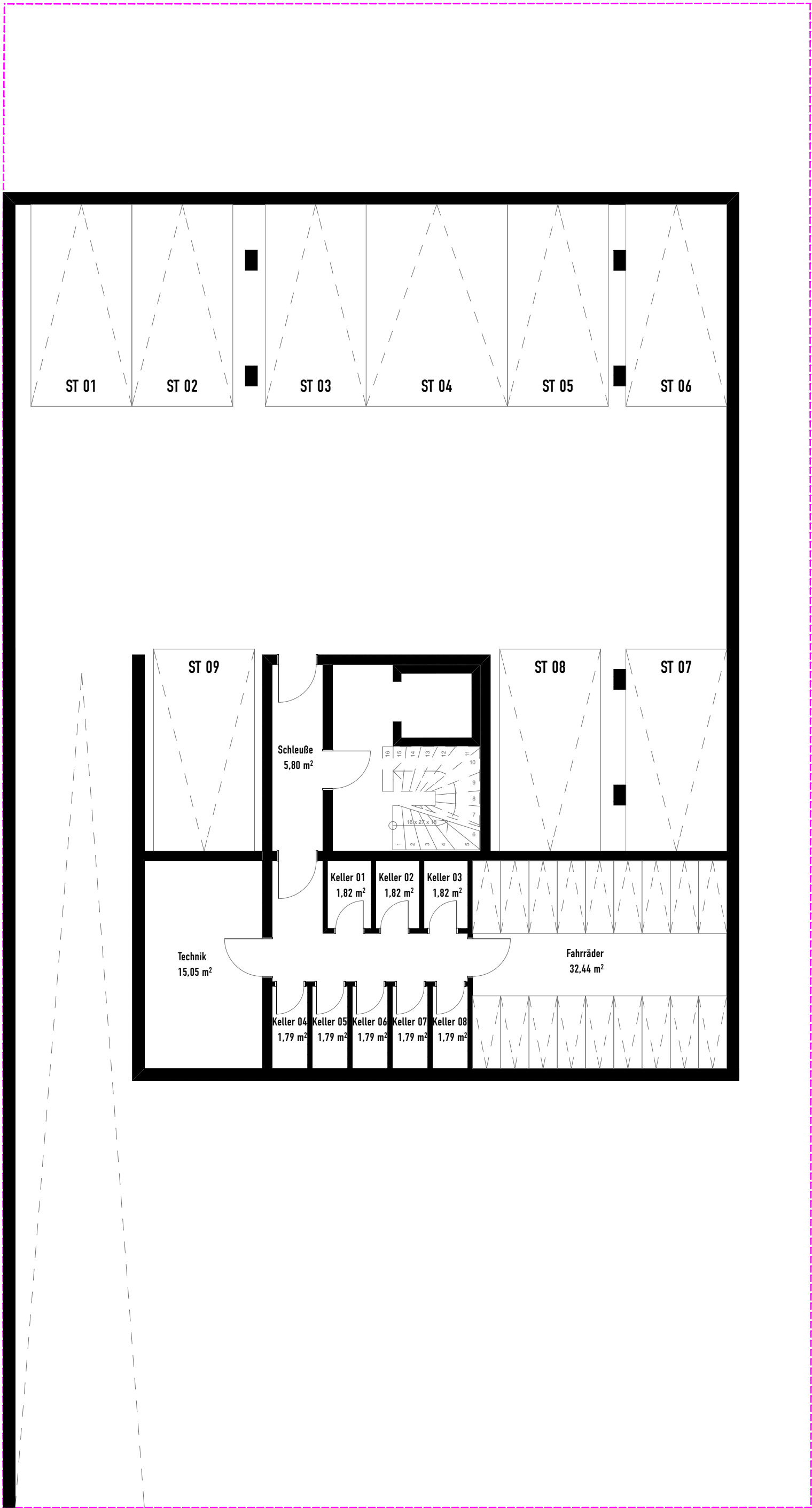
Tiefgarage 1:100
