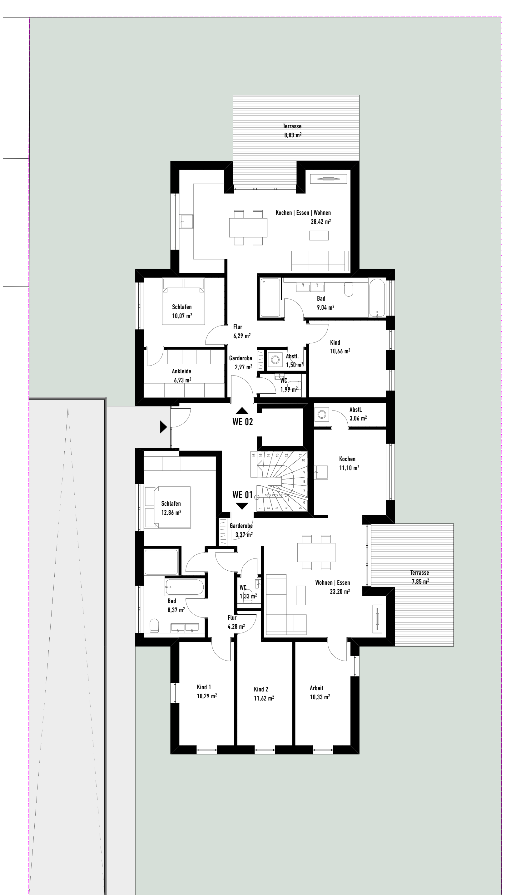
Erdgeschoss 1:100
